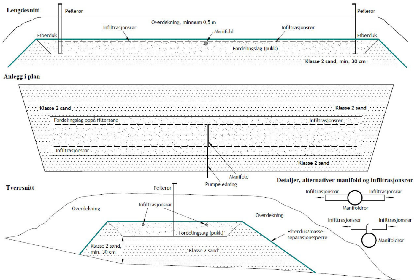
Figur 7. Prinsipptegning jordhaugfilter.
