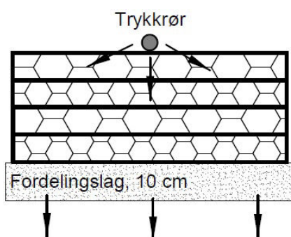
Figur 14. Prinsippskisse av biomodul.
