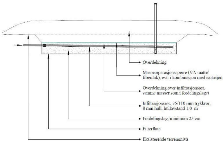
Figur 2. Prinsippskisse infiltrasjonsgrøft med selvfall.
